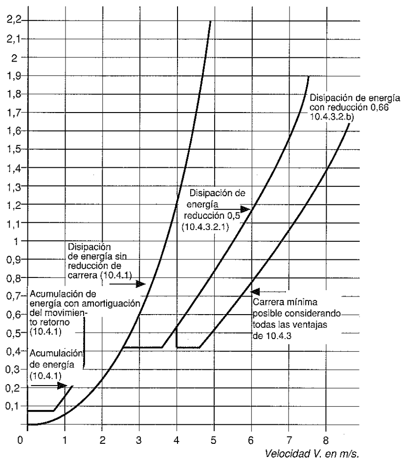
Carreras de los amortiguadores en m.
