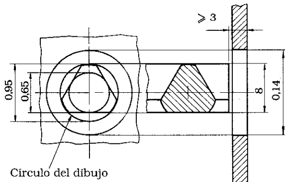
Fig. 4.—Triángulo de desenclavamiento (cotas en m.m).
